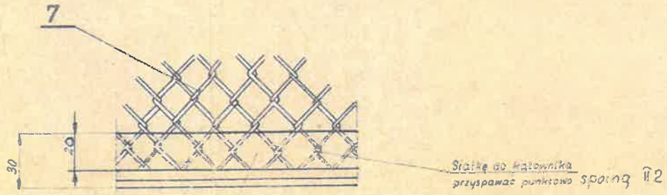
Szczegół mocowania siatki 1.2
